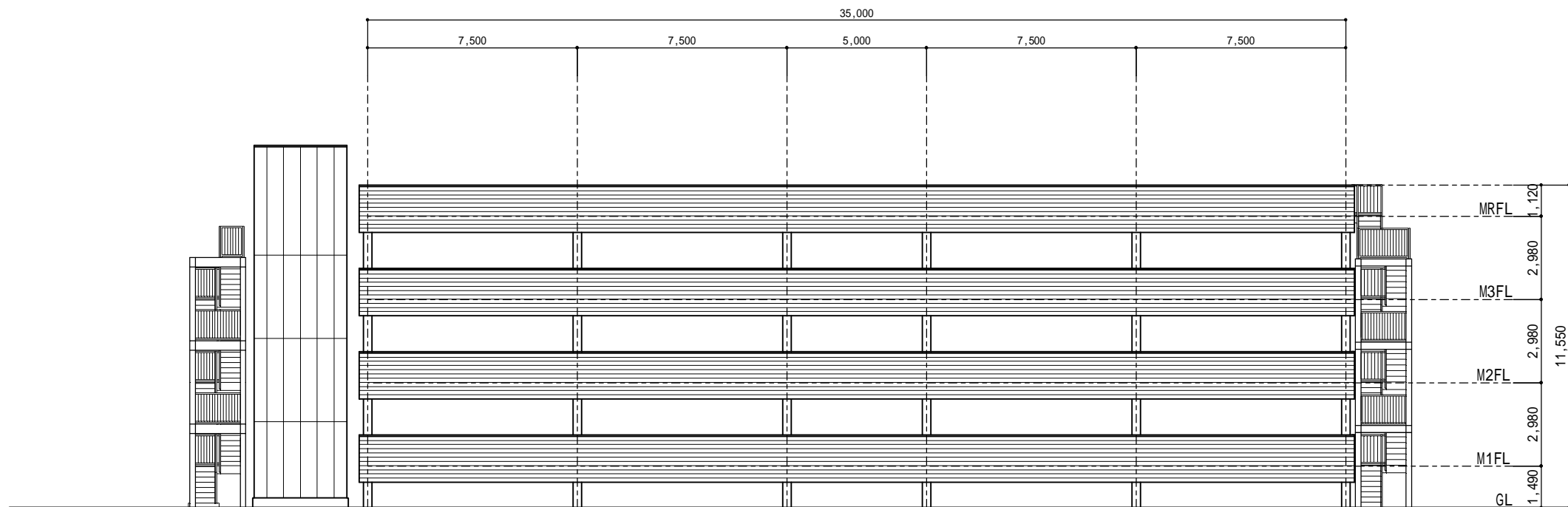
A 立面図 S = 1 : 200
