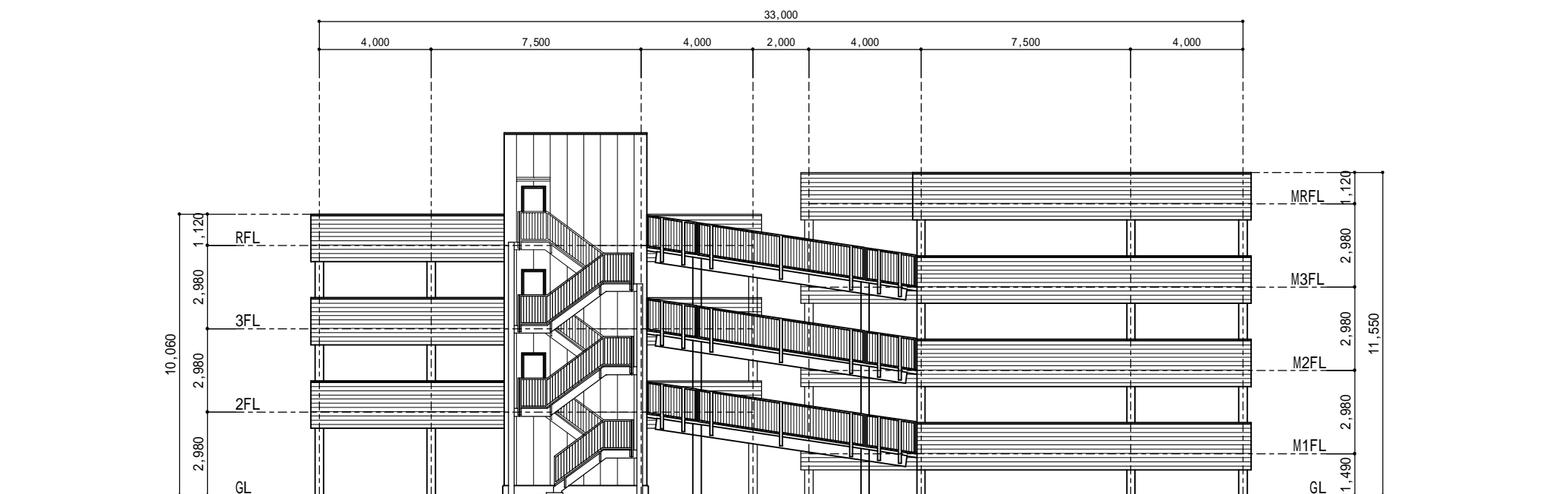
B 立面図 S = 1 : 200
