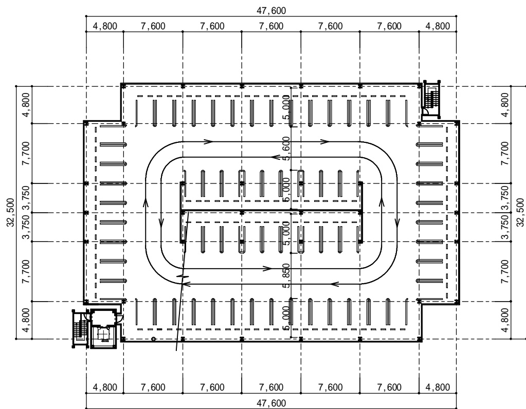
2 ~ 5階平面図 S = 1 : 500
