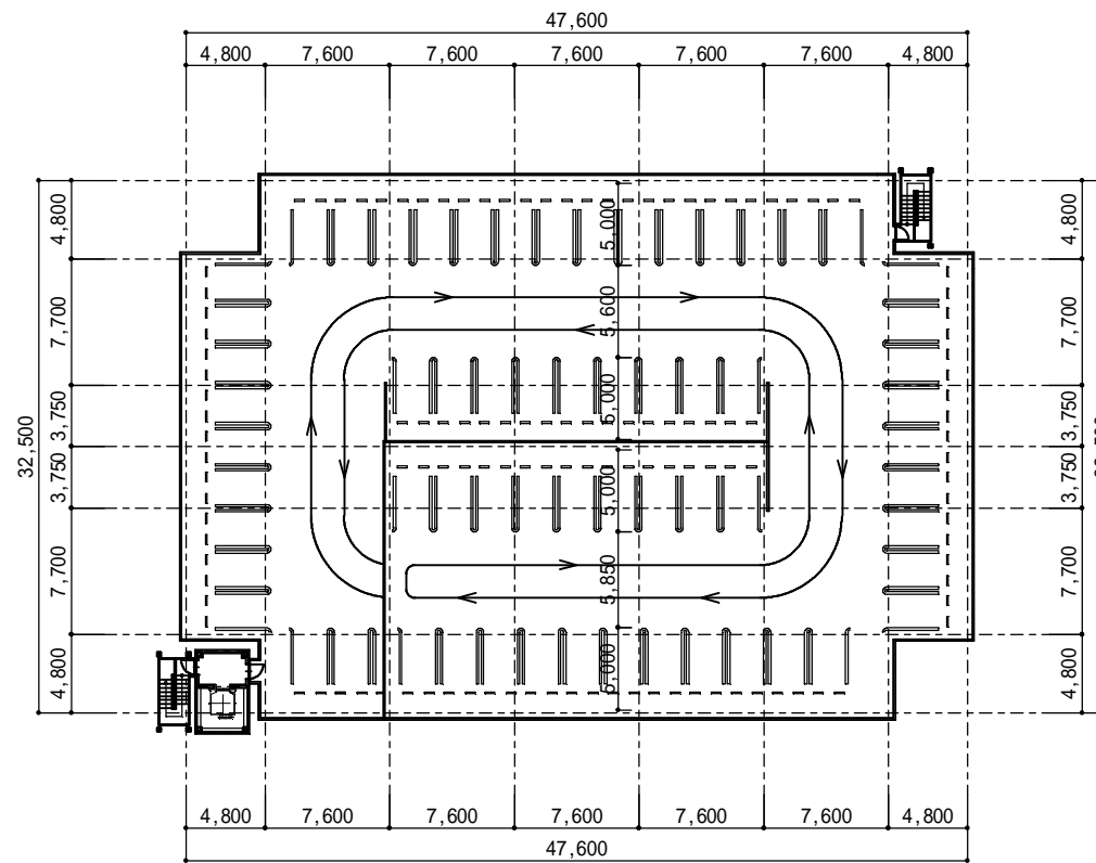
R階平面図 S = 1 : 500
