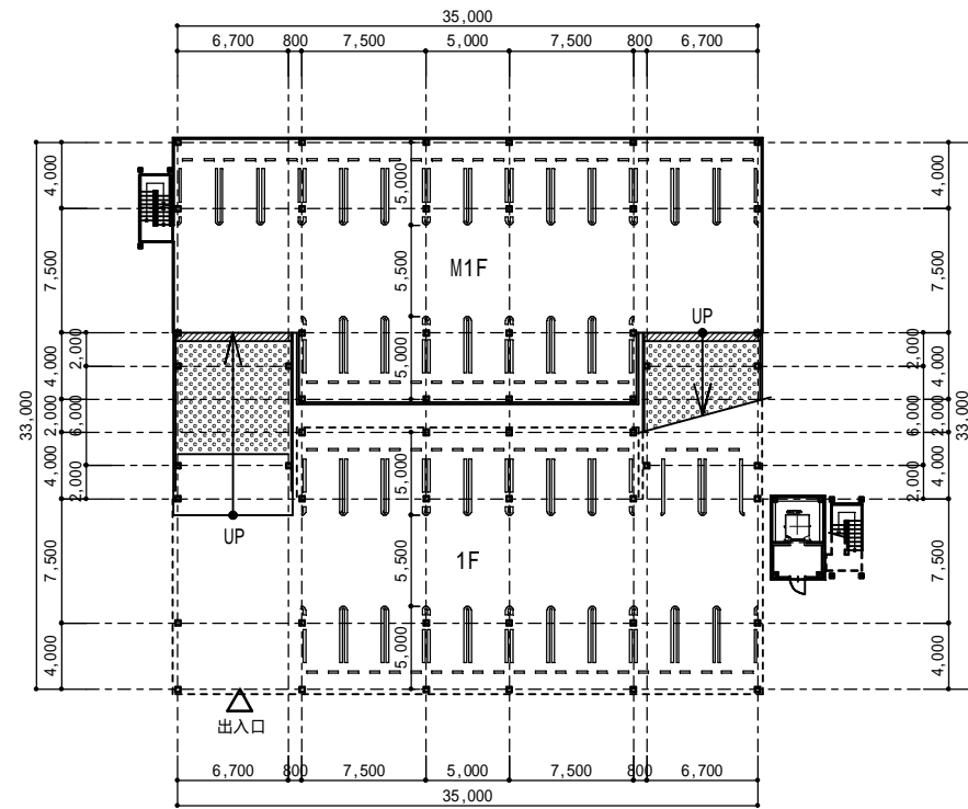
1階平面図 S = 1 : 500
