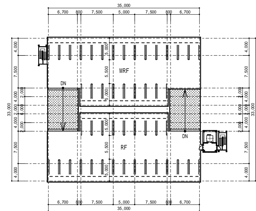
R階平面図 S = 1 : 500
