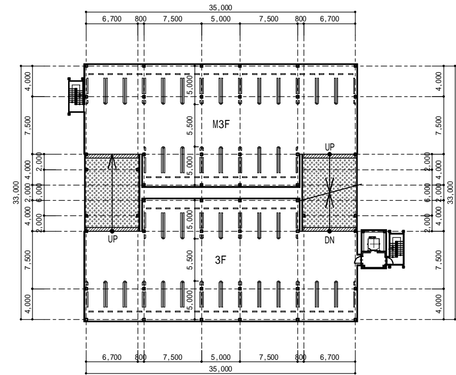
3階平面図 S = 1 : 500
