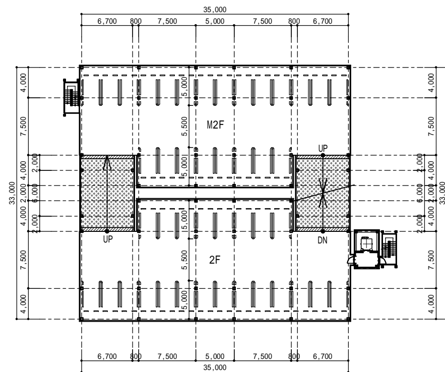
2階平面図 S = 1 : 500
